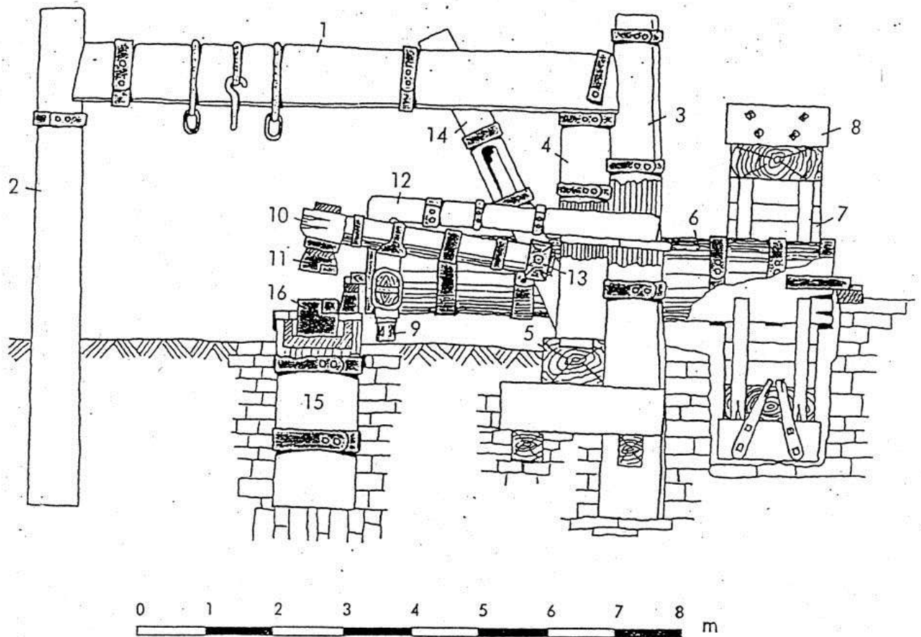
Siegerländer Aufwerfhammer zu Buschgotthardshütten bis 1908. Schematische Zeichnung von Fr. Oehler 1948
